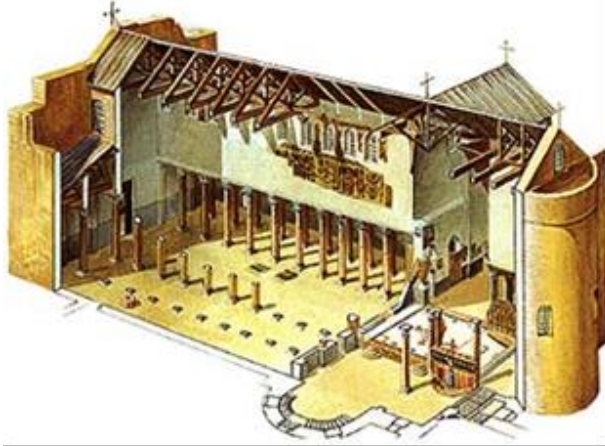
شكل (10) رسم توضيحي لعمارة كنيسة المهد الكبرى - بيت لحم
