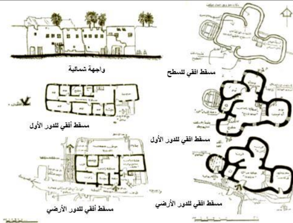
بعض النماذج للبيت السيوي التقليدي ويتضح استخدام نظام البناء الحوائط الحاملة
