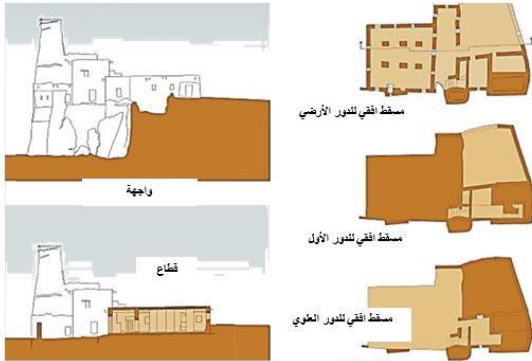
المساقط الأفقية والواجهات والقطاعات لمسجد العتيق بعد الترميم والإرتقاء
