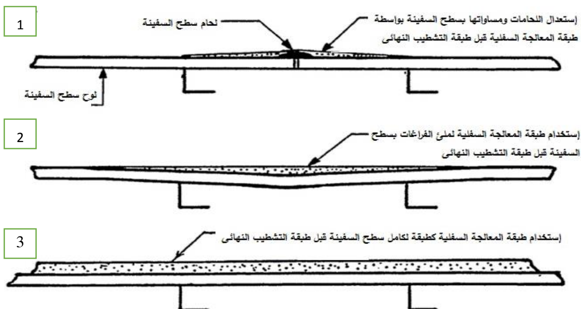
شكل رقم 11 يوضح الأغراض المتعددة لإستخدام اللاتكس فالرقم (1) يبين إستخدام اللاتكس لإستعداد أو تسوية اللحات مع السطح والرقم (2) يوضح إستخدام اللاتكس كمادة مالئة لملو المناطق المنخفضة والرقم (3) يوضح إستخدام اللاتكس كطبقة تجهيز تحت الطبقة النهائية
