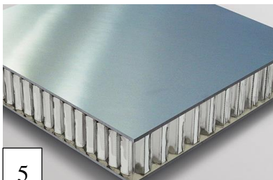
شكل رقم (7) يوضح الأنواع المختلفة للنواة الأساسية لألواح الساندوتش (1 مواد رغوية - 2 فوم - 3 صفائح مموجة - 4 خلية نحل هانى كومب) ورقية - 5 خلية نحل هانى كومب) من الألومنيوم - 6 الخشب
